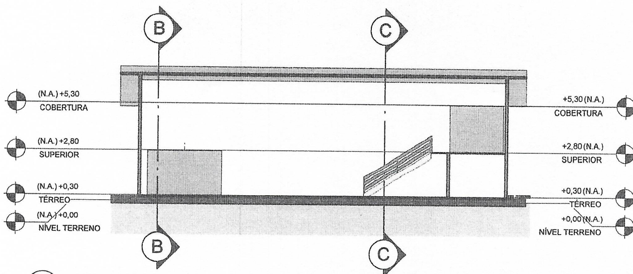
2 Corte DD ESCALA 1 : 200
