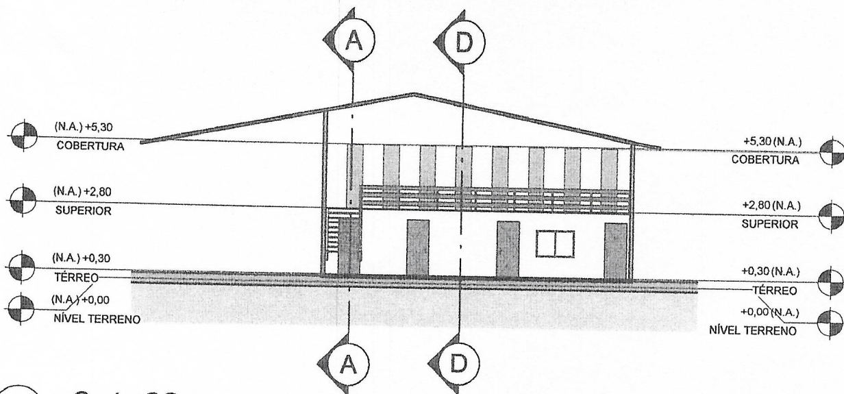
1 Corte CC ESCALA 1 : 200
